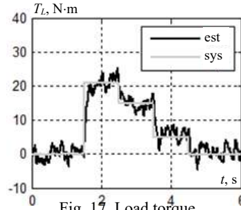
Fig. 17. Load torque
