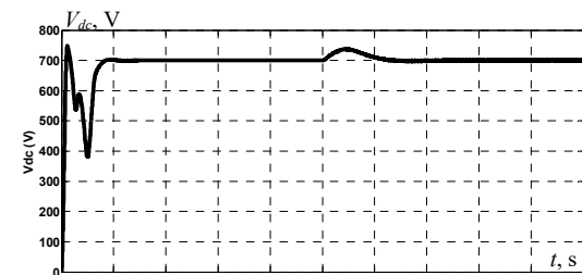
Fig. 19. DC voltage
