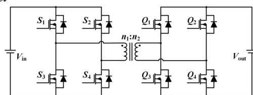
Fig. 4. DAB DC-DC converter
